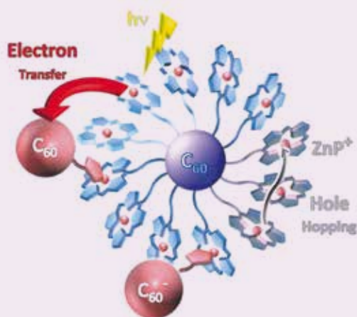
Fig. 2 Rappresentazione schematica di un sistema supramolecolare autoassemblato, costituito da 12 unità porfiriniche e due tipi diversi di fullerene, nel quale avvengono alcuni processi fondamentali della fotosintesi artificiale: raccolta dell'energia luminosa, separazione di carica, hole hopping
